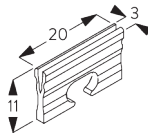
SG 11237 Wedge
